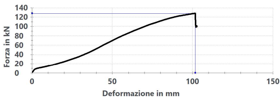
Figura 1 - Grafico forza – corsa traversa
