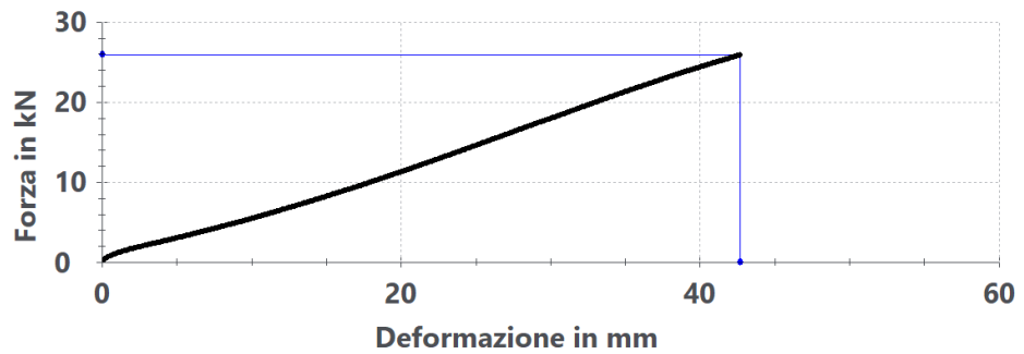
Figura 1 - Grafico forza – corsa traversa
